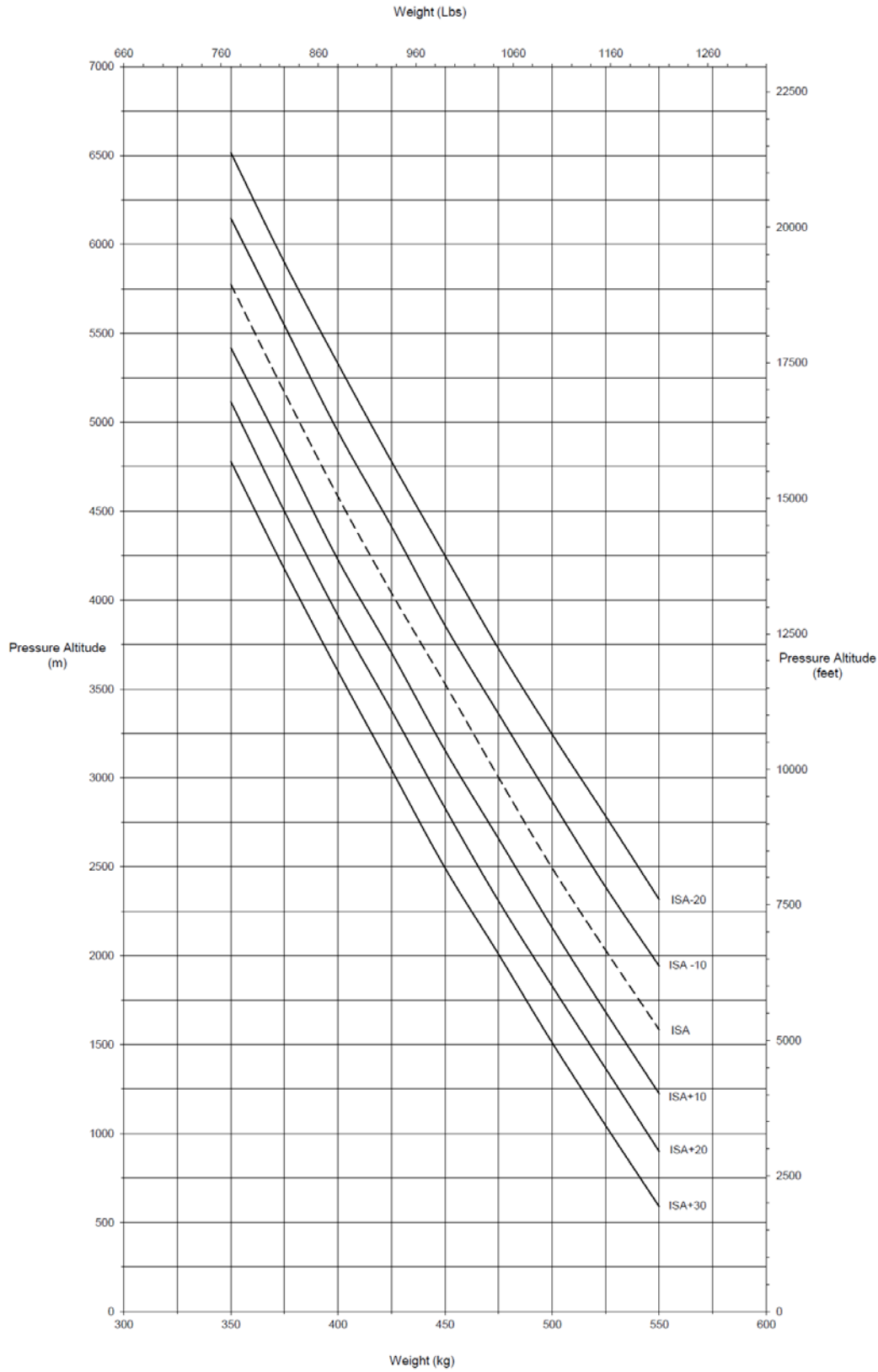
Hovering ceiling - OGE
