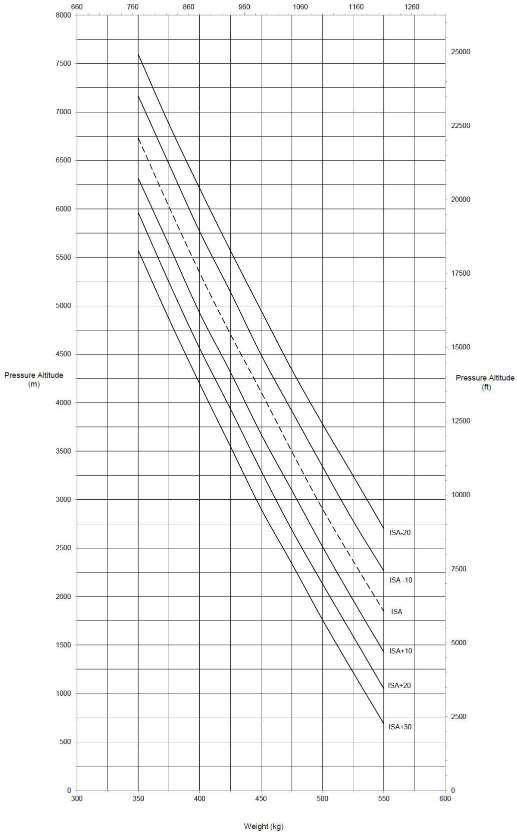
Hovering ceiling - IGE
